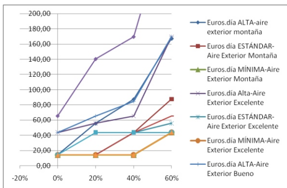
Figura 3: Ahorro económico en función de la calidad del aire exterior e interior.
