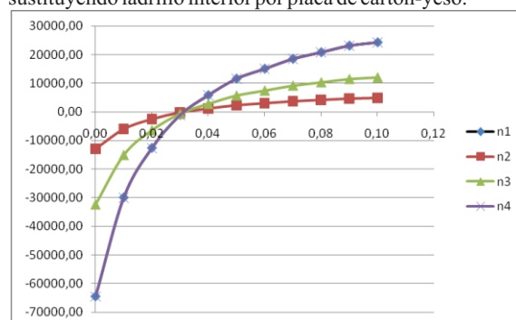
Figura 2: Ahorro económico en 10,25 y 50 años sustituyendo la cámara del cerramiento por aislante.
